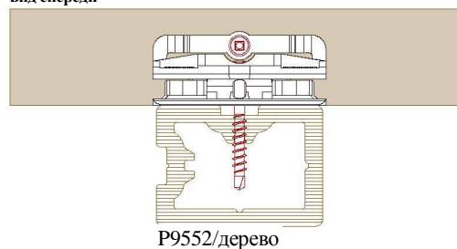
вид спереди
